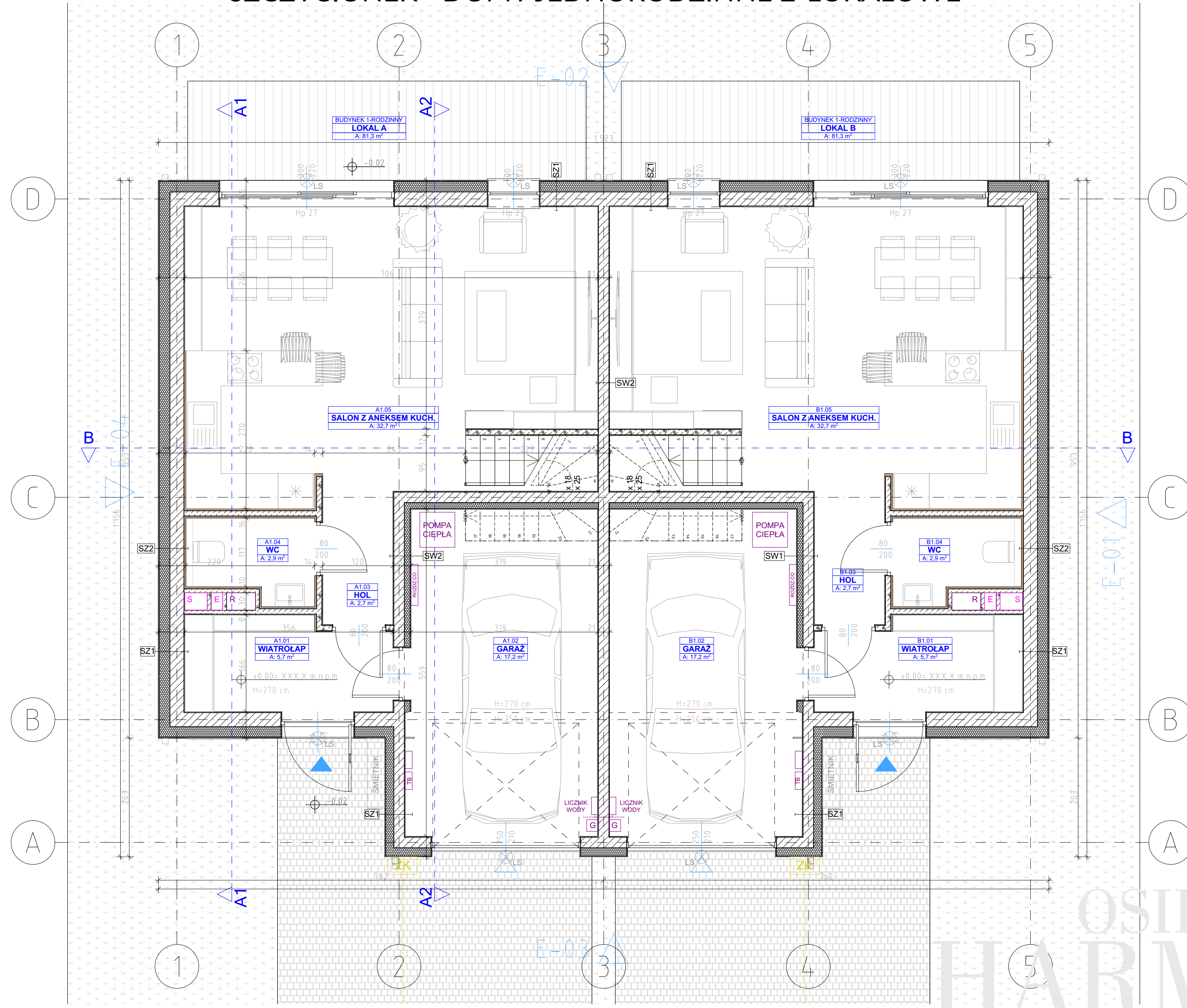
RZUT PARTERU
