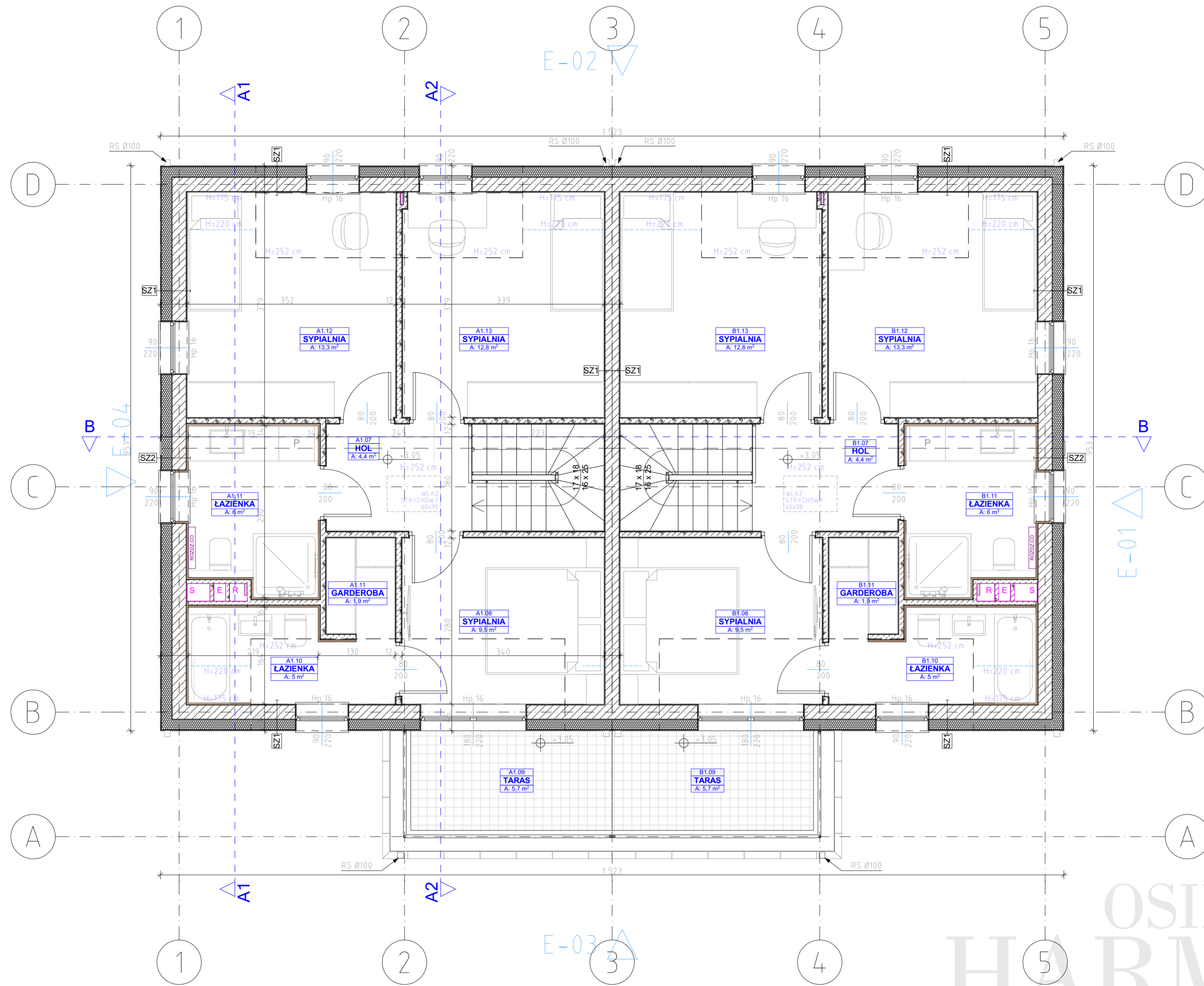
RZUT PODDASZA
